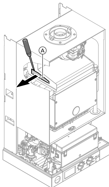
Ⓐ Tablă ștanțată
